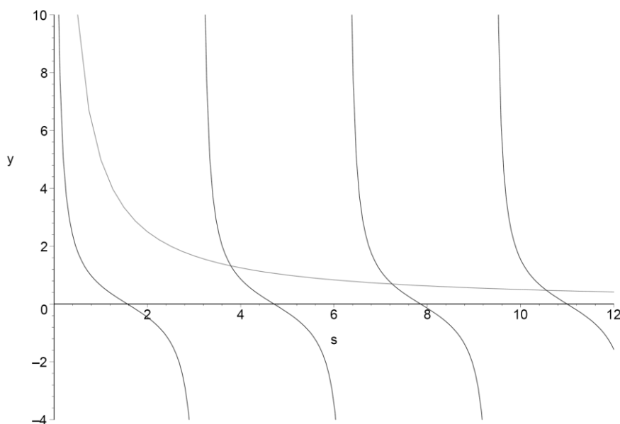
Рис. 1. Спектр краевой задачи при \beta_0 = 0
